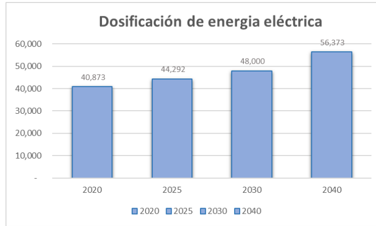
Gráfica 4.3. 1 Dosificación de energía eléctrica
