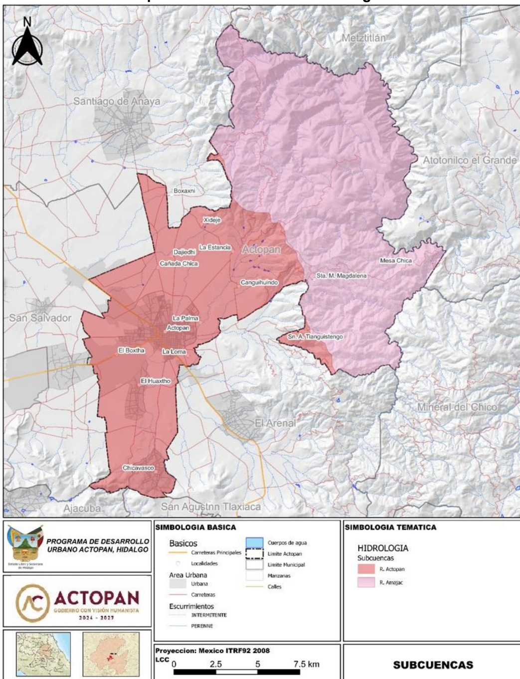
Mapa 2.2.1.7. Subcuencas Hidrológicas.
