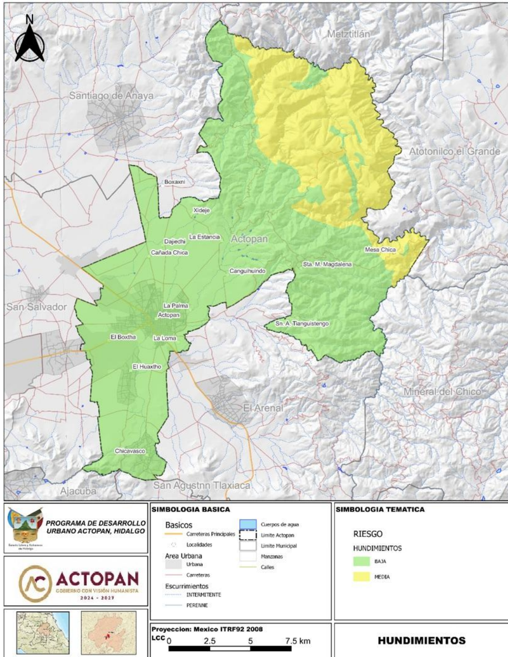
Mapa 2.2.3.1.3 Hundimientos
