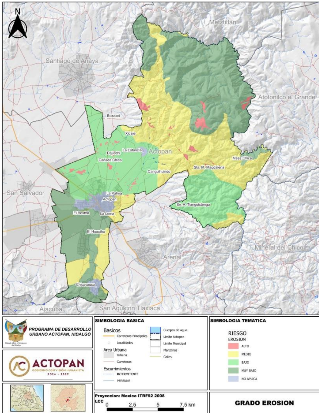
Mapa 2.2.3.3.1. Grado de riesgo del fenómeno de erosión dentro del Municipio.
