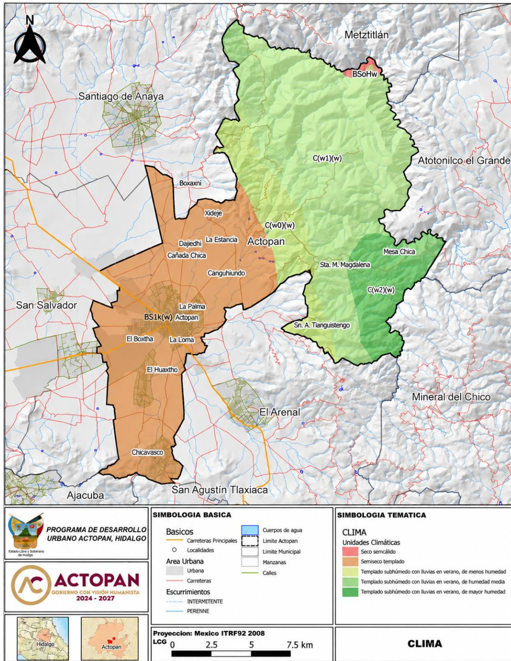
Mapa 2.2.1.3. Unidades Climáticas
