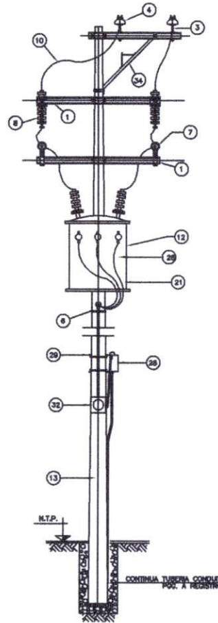
SECCION B - B SUBESTACION EN POSTE TR-3
