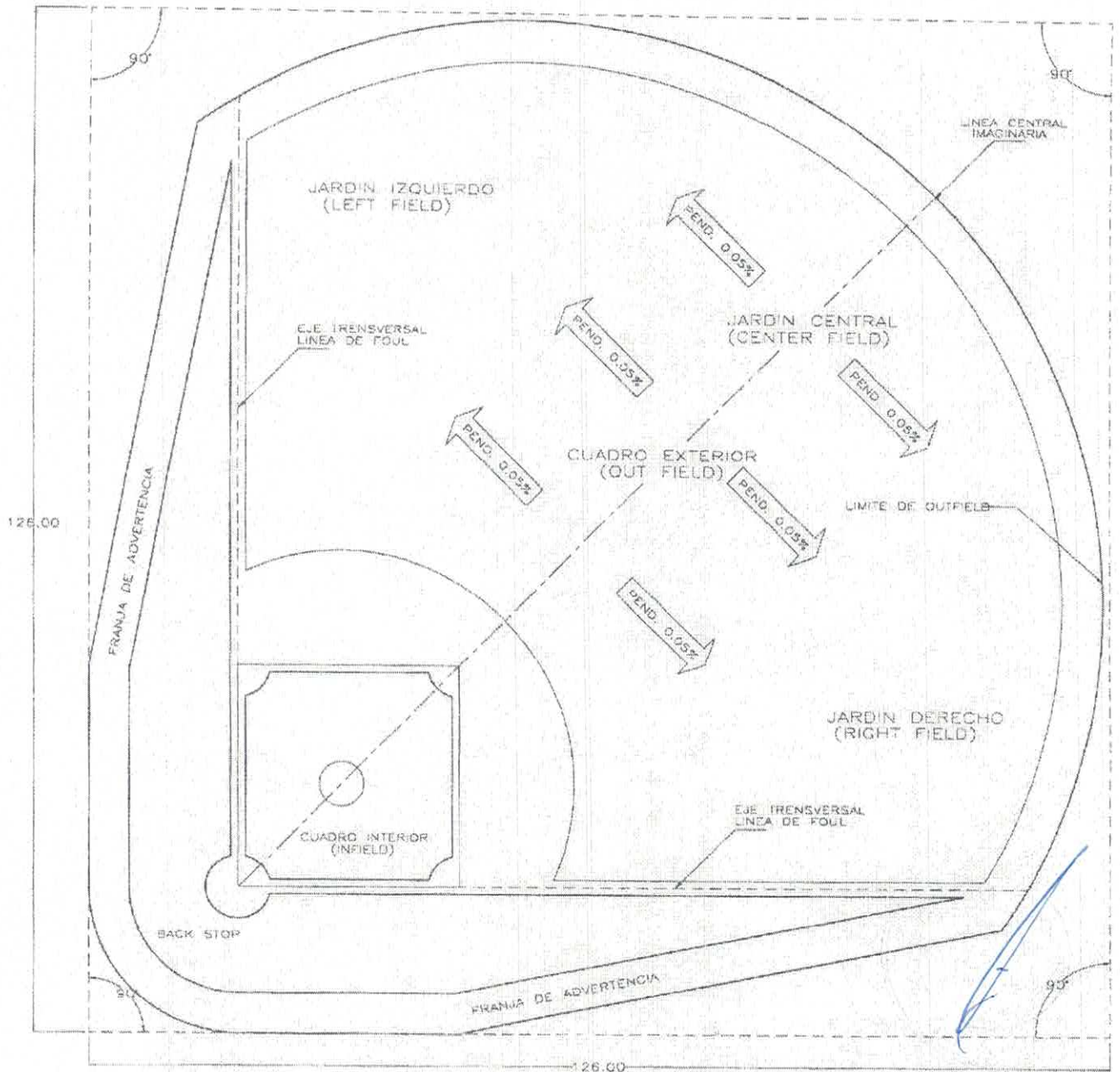
2.01 PLANTA
